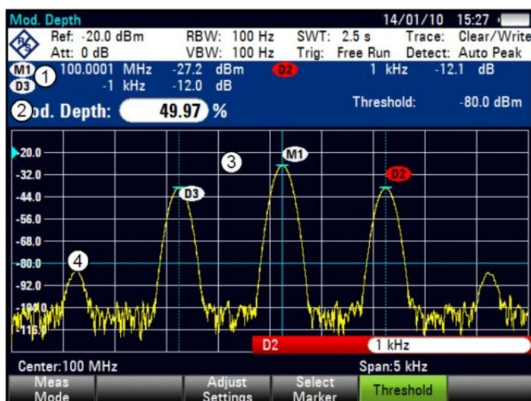
Рисунок 8.9 – Вид экрана при измерении коэффициента модуляции АМ-сигнала
