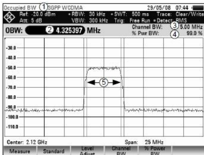
Рисунок 8.4 – Вид экрана при измерении занимаемой полосы частот
