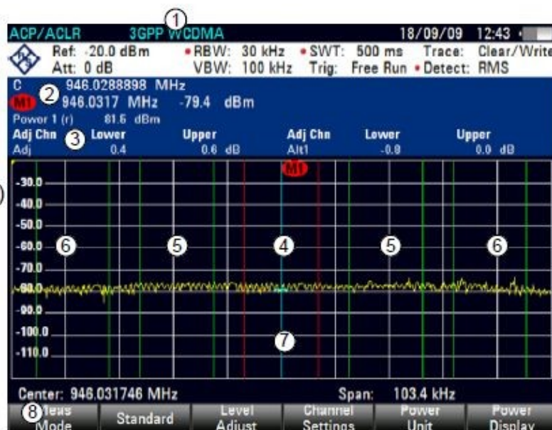
Рисунок 8.6 – Вид экрана при измерении мощности в соседнем канале
