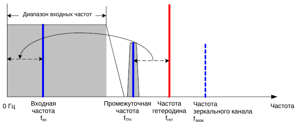
Рисунок 8.14 – Преобразование частот в анализаторе спектра
