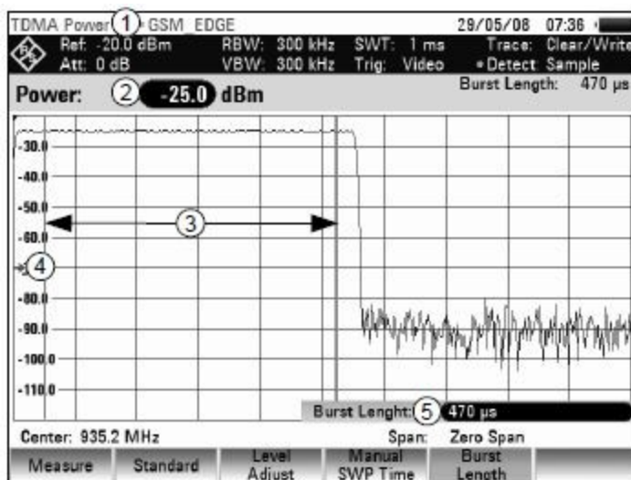
Рисунок 8.5 – Вид экрана при измерении мощности TDMA-сигналов
