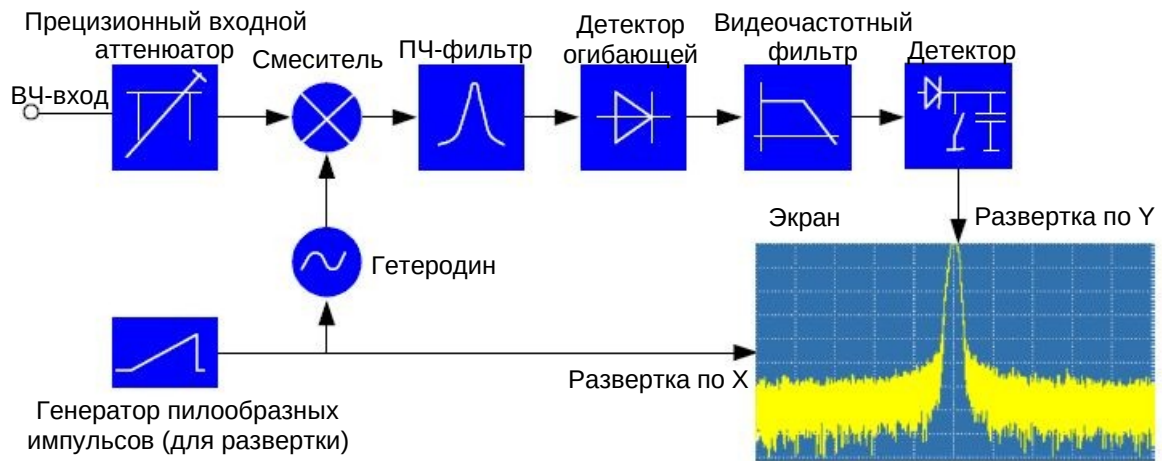
Рисунок 8.13 – Структурная схема анализатора спектра
