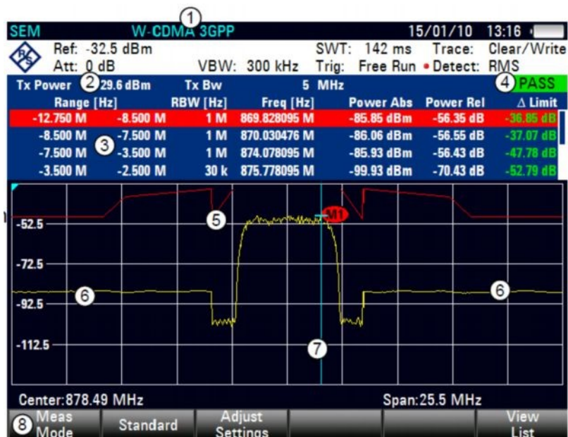
Рисунок 8.7 – Вид экрана при измерении спектральной маски излучения
