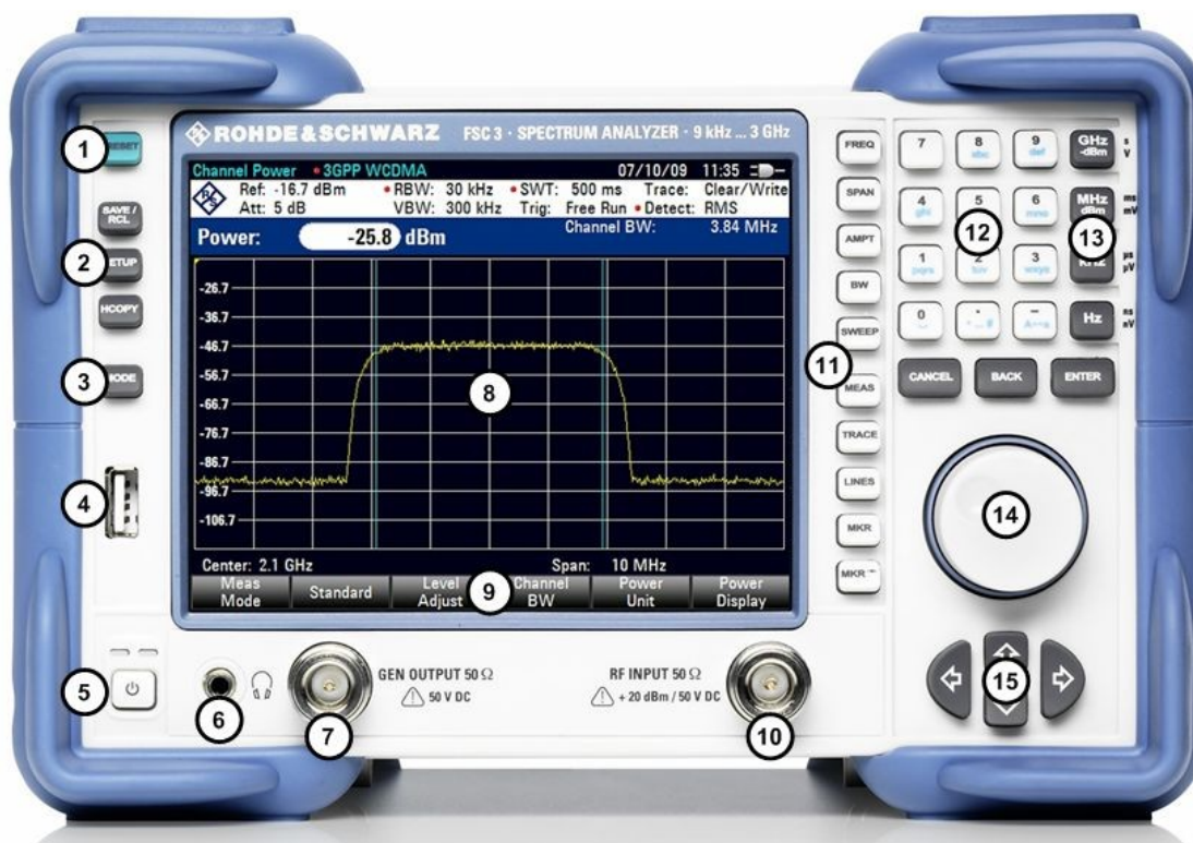
Рисунок 7.1 – Анализатор спектра R&S FSC. Вид спереди.
