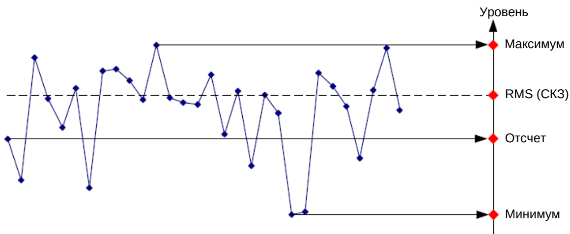
Рисунок 8.17 – Пояснение принципа работы детекторов
