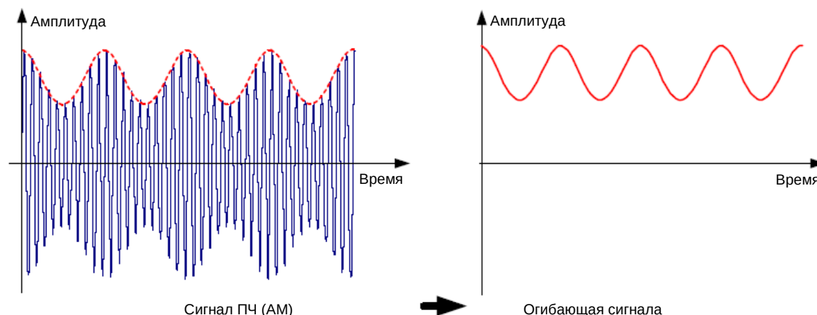
Рисунок 8.15 – Выделение огибающей амплитудно-модулированного сигнала
