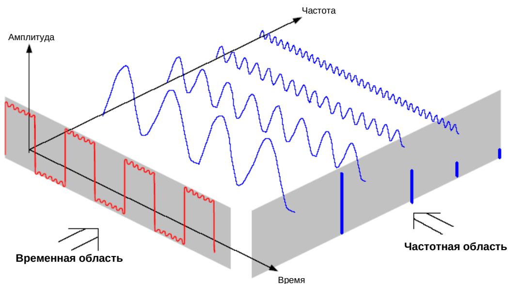
Рисунок 8.12 – Анализ сигнала в частотной и временной области
