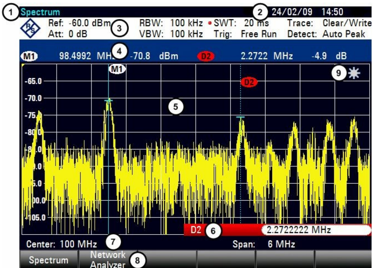
Рисунок 7.2 – Основные элементы экрана анализатора спектра R&S FSC
