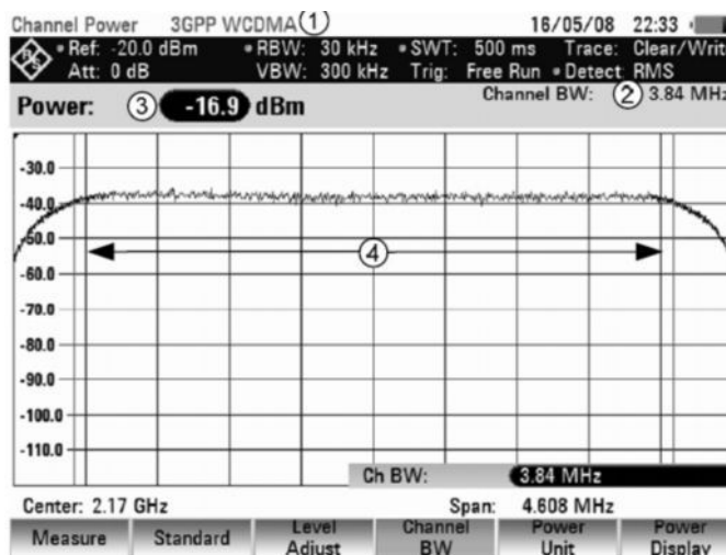
Рисунок 8.3 – Вид экрана при измерении мощности в канале
