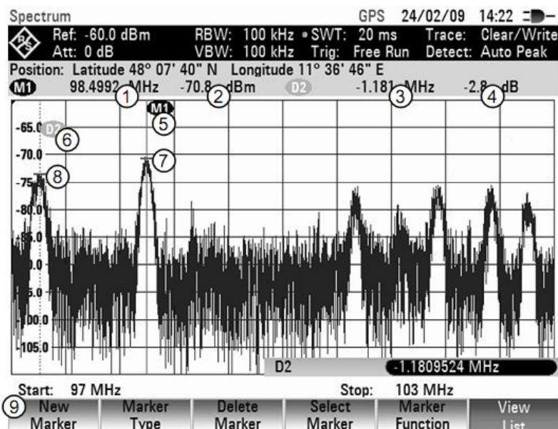
Рисунок 8.2 – Вид экрана в режиме использования маркера
