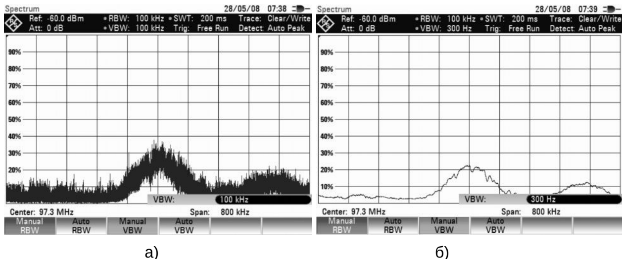
Рисунок 8.16 – Влияние полосы видеофильтра на спектрограмму сигнала
