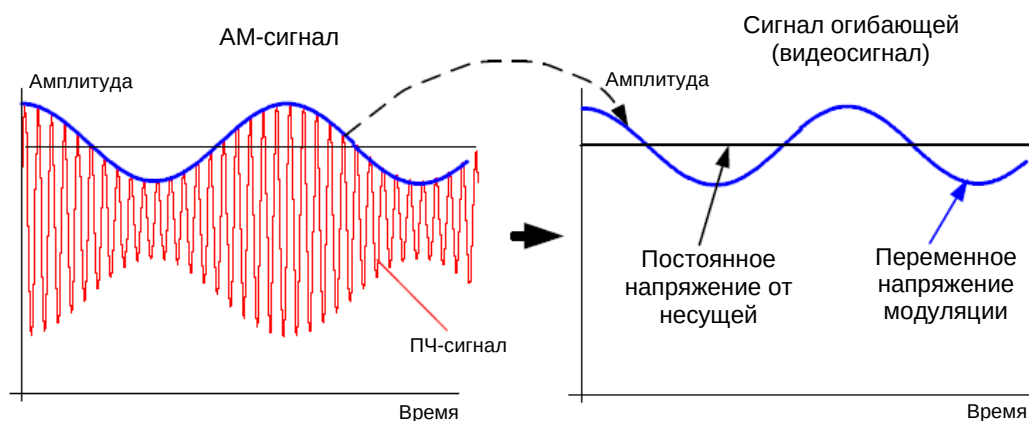
Рисунок 8.1 – Сигнал огибающей (видеосигнал)
