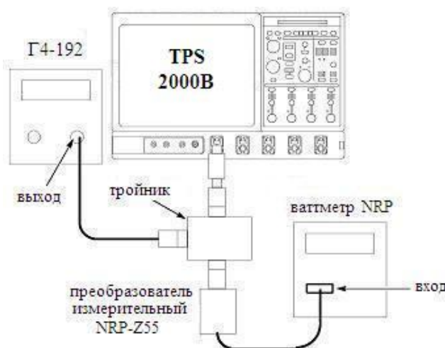
Рисунок 26 - Схема определения полосы пропускания
