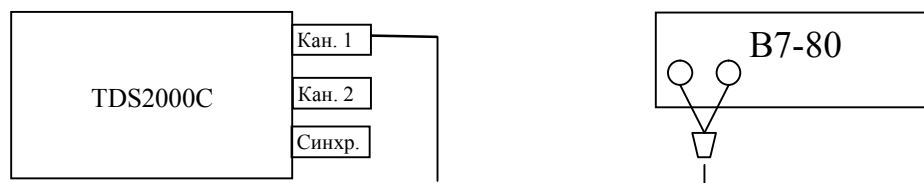
Рисунок 4- Схема определения входного сопротивления
