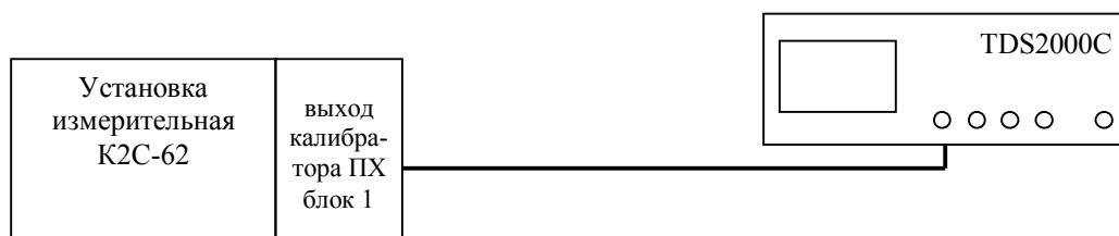
Рисунок 2- Схема определения полосы пропускания осциллографа
